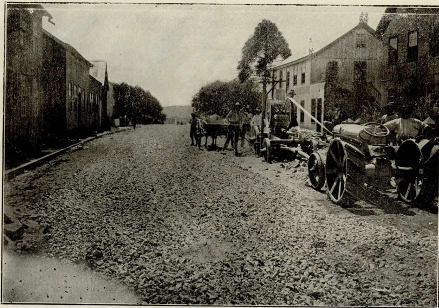
O trabalho de macadamisação das ruas distantes do local da pedreira è feito no proprio lceal, aproveitando um tractor e uma britadeira movel (Avenida Rio Branco)
